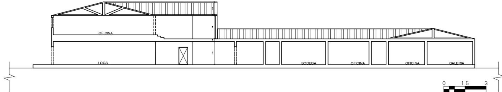
Corte longitudinal
